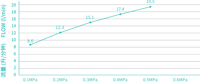
流量图 FLOW RATE CHART
